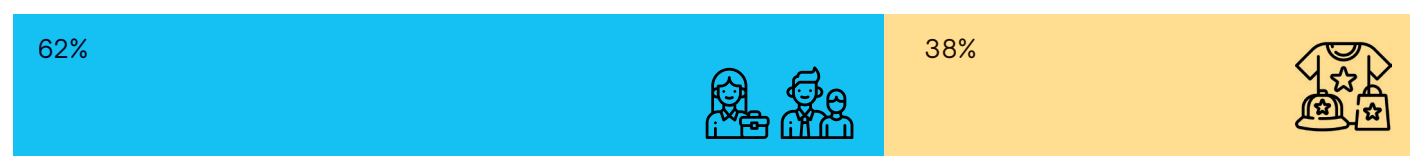
Consommation d'énergie primaire pour le secteur du transport sur le territoire de la CCDB
