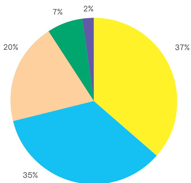
Émission de gaz à effet de serre par secteur sur le territoire de la CCDB en CO 2 équivalent
