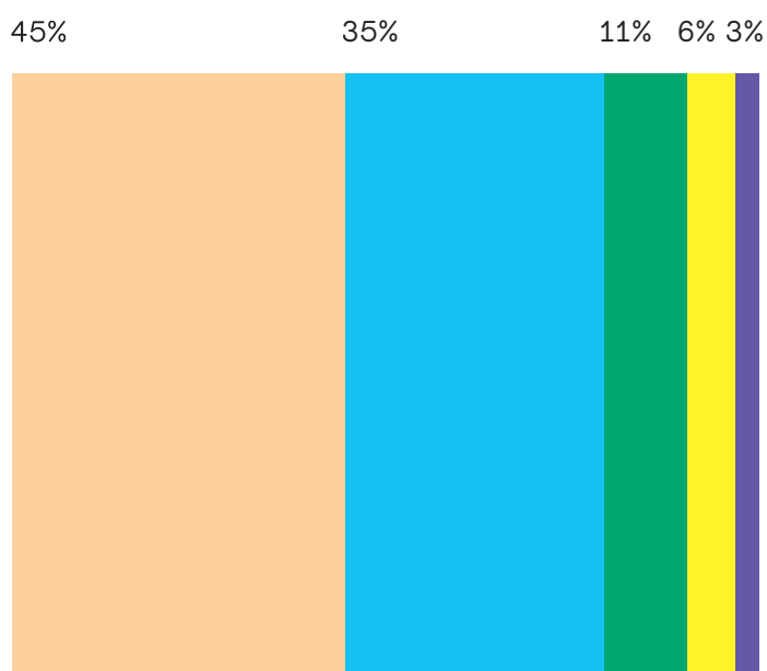
Consommation d'énergie primaire par secteur sur le territoire de la CCDB
