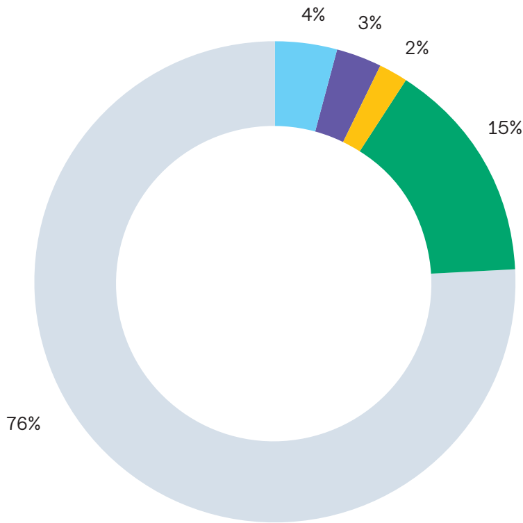
Répartition de la production d'énergie de la CCDB par type
